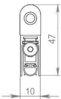
Автоматический порог врезной
