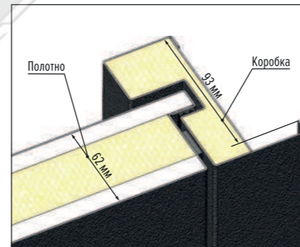
EI-60 (сплошной противосъем)
