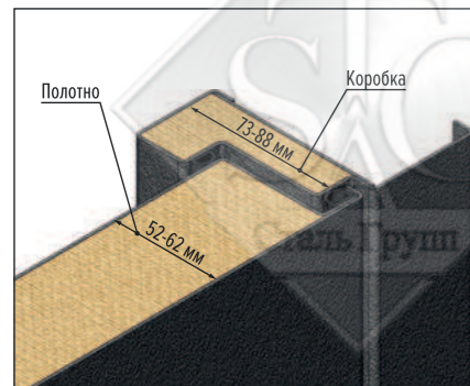
Техническая двойной контур
