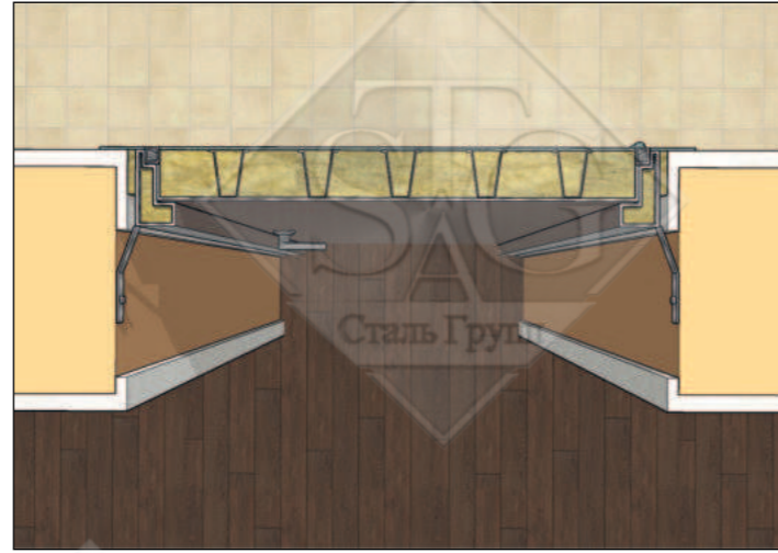
Вид изнутри сверху
