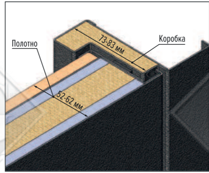
EI-60 (МДФ панель внутри)
