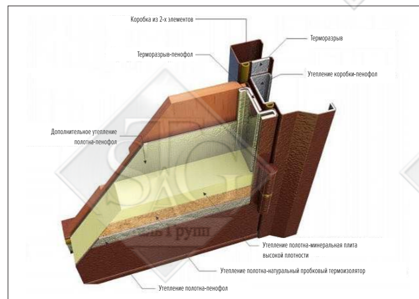
Конструкция двери с терморазрывом в разрезе
