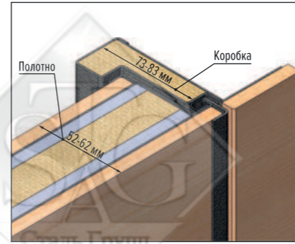
EI-60 (МДФ панель с двух сторон)
