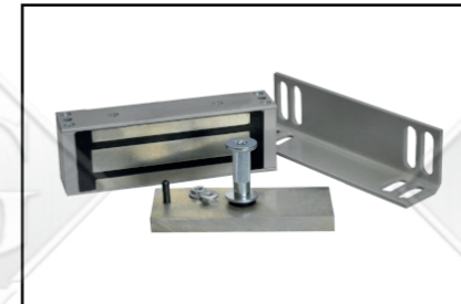
Электромагнитный замок M1-300
