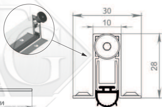
Автоматический порог накладной
