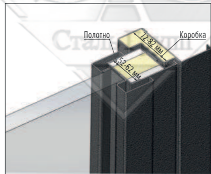
EIW-60 (остекление более 25%)
