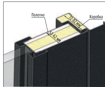
EI-60 (остекление до 25%)
