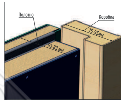
EI-60 (наружное полотно)
